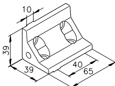
Angle E65s 82.40.0744
