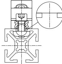
Angle M25
