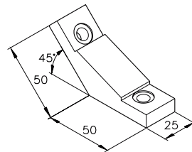
Angle M25 82.11.4001
