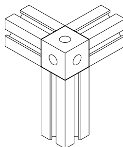
Corner block 5 79.01.0005
