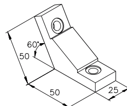
Angle N25 82.12.4001
