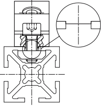
Angle M25s
