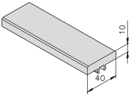
Wear strip mk 1040.02 21.02.2000
