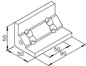
Angle B90 82.05.0022 T82.05.0022*
