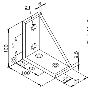
Angle bracket 4 31.00.0004
