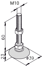
Levelling foot ø 45 M10 B67.02.057
